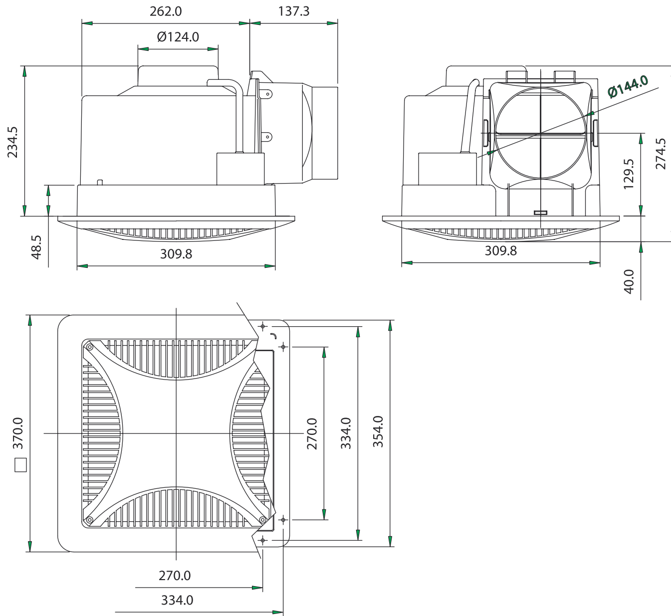
外觀尺寸圖 (單位: mm)
